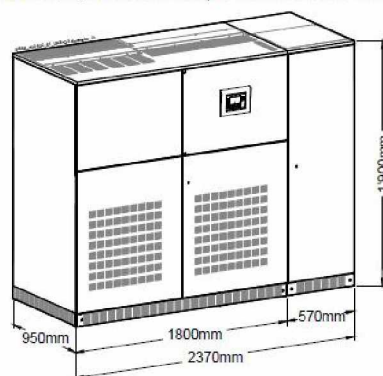
Размеры (ШхГхВ): 2370 x 950 x 1900 мм
